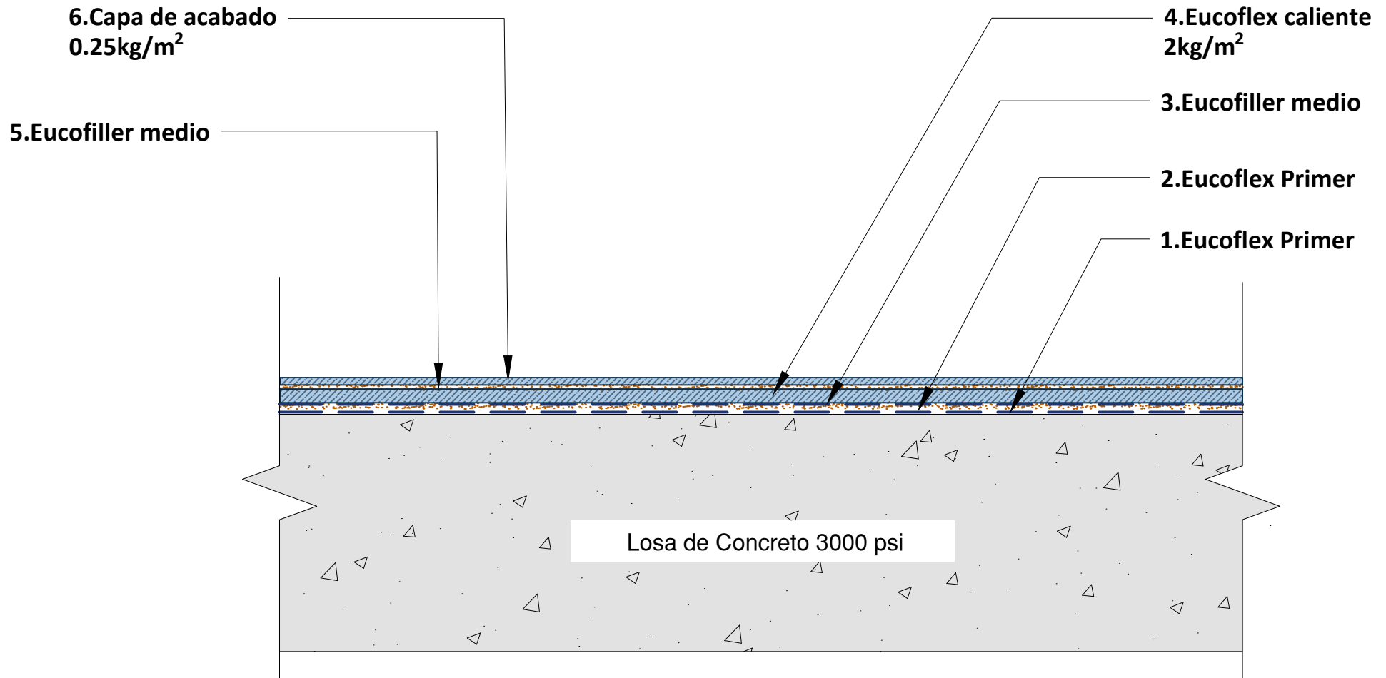
DETALLE SISTEMA EUCOFLEX CALIENTE
