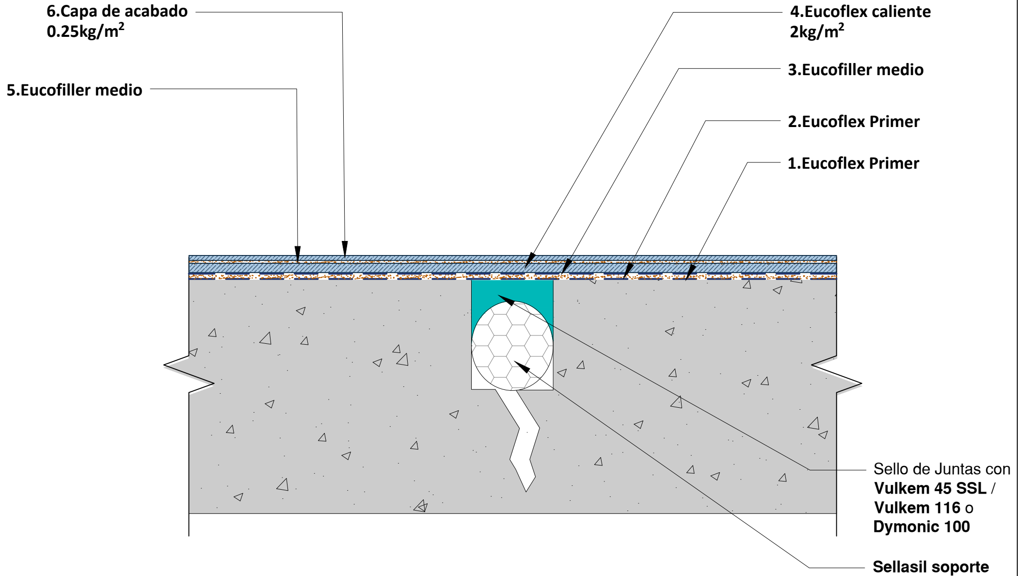
TRATAMIENTO DE FISURAS MAYORES A 1.6 MM / SELLO DE JUNTAS DE DILATACIÓN
